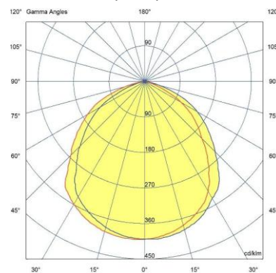
Светло разпределение
