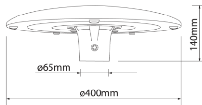
Размери
